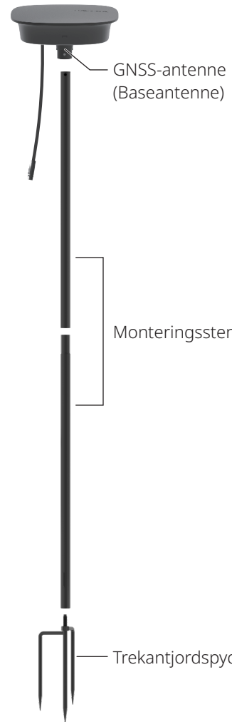
RTK-referansestasjon
