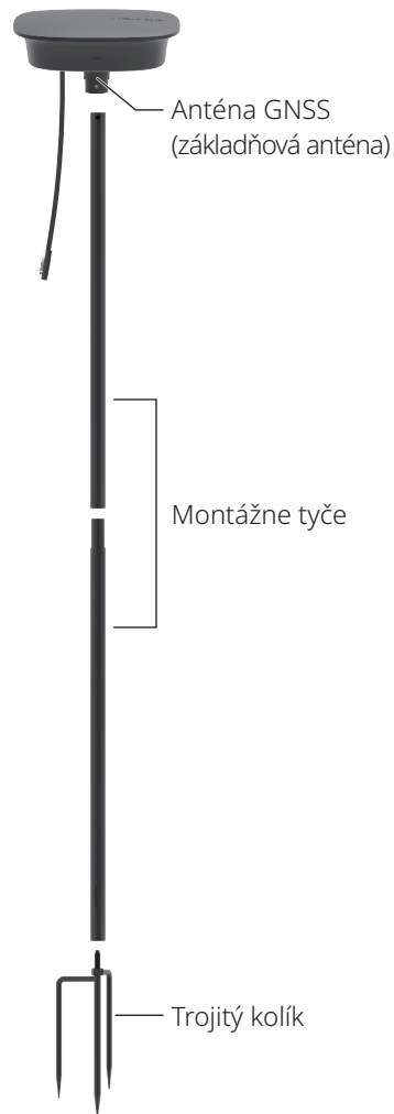
Referenčná stanica RTK
