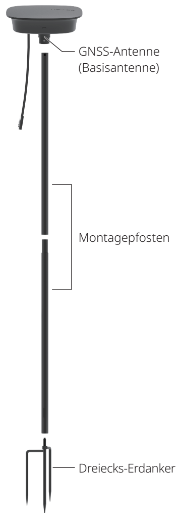
RTK-Referenzstation
