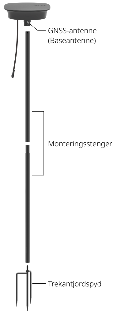
RTK-referansestasjon
