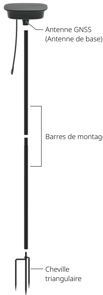
Station de référence RTK
